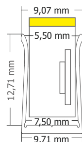
Montage im Profil mounting in profile
